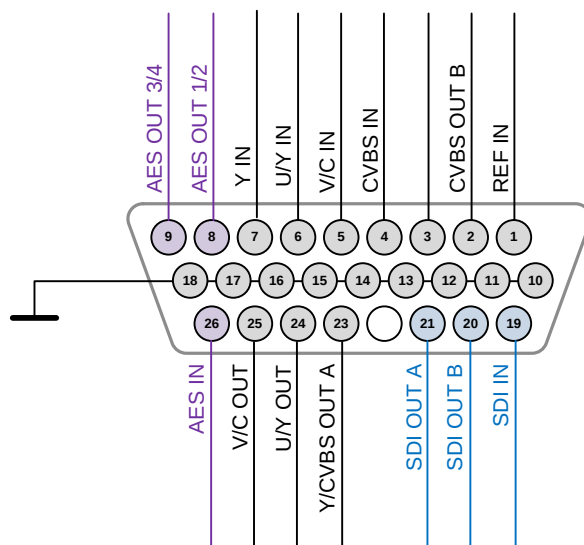
Разъем ВИДЕО/AES (верхний) вид со стороны распайки кабелей
