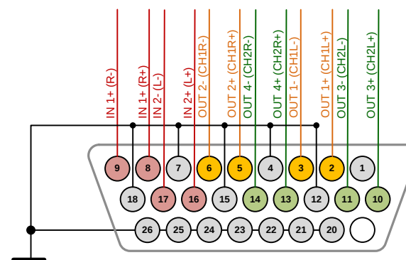
Разъем ANALOG AUDIO (нижний) вид со стороны распайки кабелей
